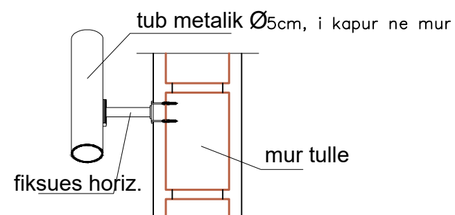
DETAJ 1 SH 1:10
