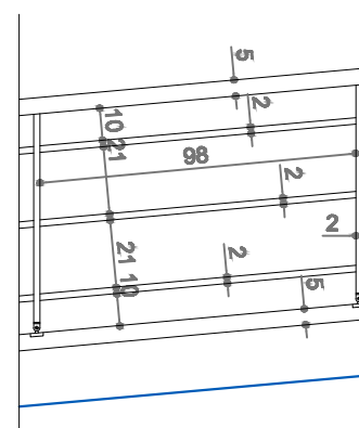
DETAJ 2 SH 1:10
