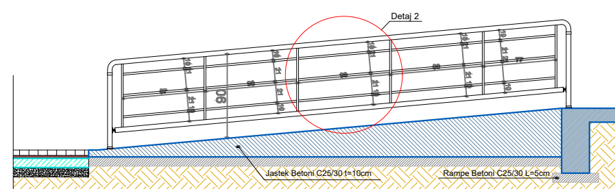
DETAJ I RAMPES SH 1:25
